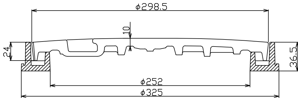
A - A' 断面
