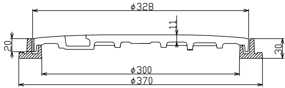
A - A' 断面図
