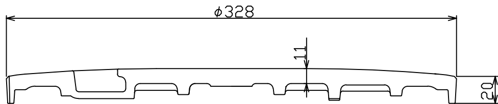
A - A' 断面図
