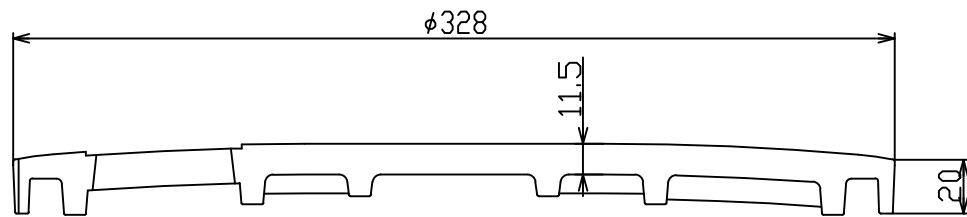
A-A' 断面図
