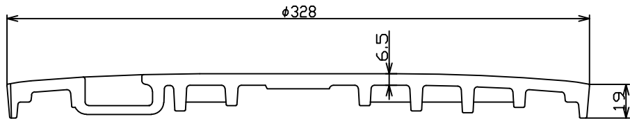
A-A' 断面図
