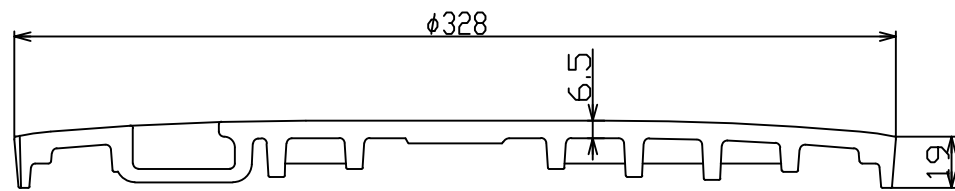
A-A' 断面図
