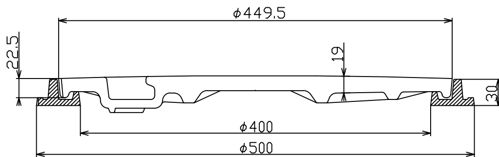
A-A' 断面図
