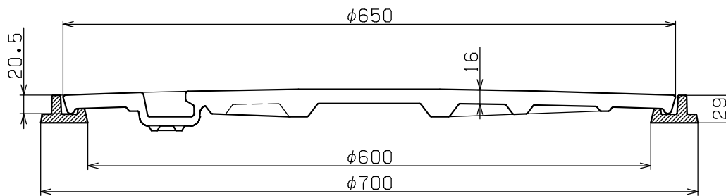
A-A' 断面図
