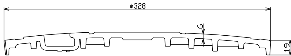
A-A' 断面図
