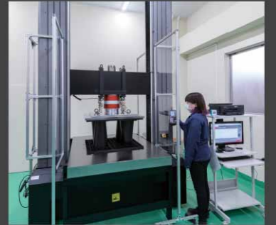
▶ インストロン社製600kN試験機
